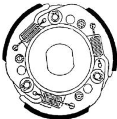
Girante frizione con molle standard per campane diam. 105 (Motori Minarelli prima del 1997)
