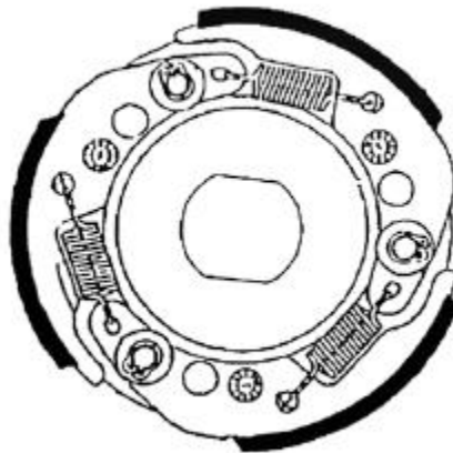
Girante frizione con molle standard per campane diam. 107 (Motori Piaggio All Models e Motori Minarelli dopo il 1997)
